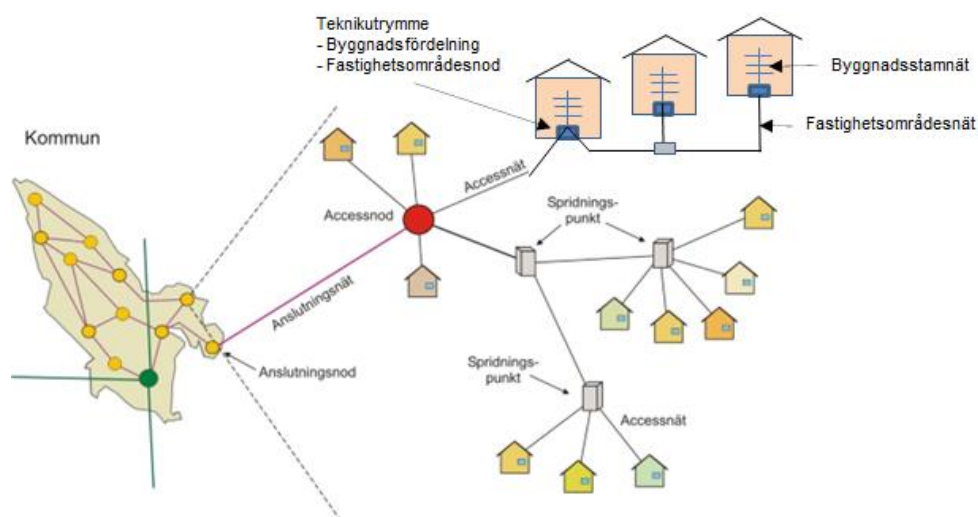
Bild 4. Anslutning av Fastighetsnät till lokal infrastruktur
