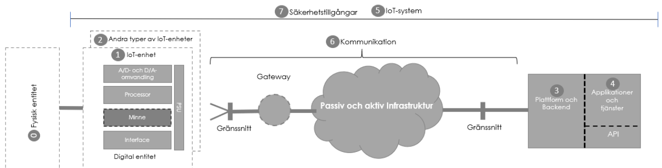
Bild: Konceptuellt IoT-system
